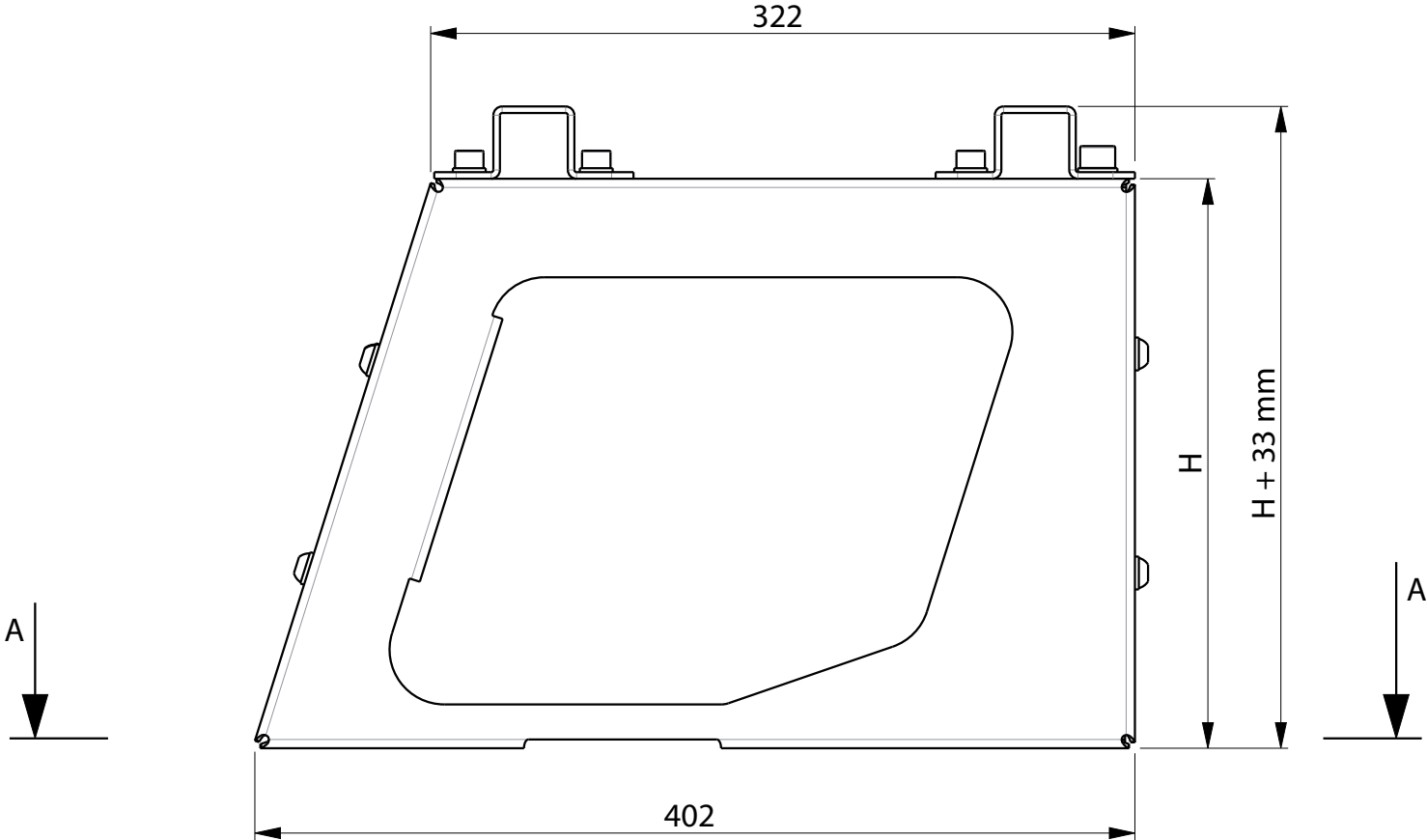
Seitenansicht
